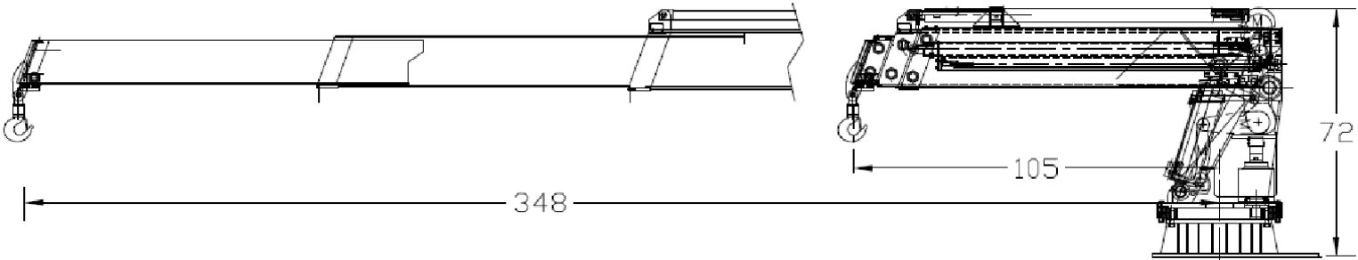
OPTIONAL ARA 309 CRANE 6000 LB @ 29'
